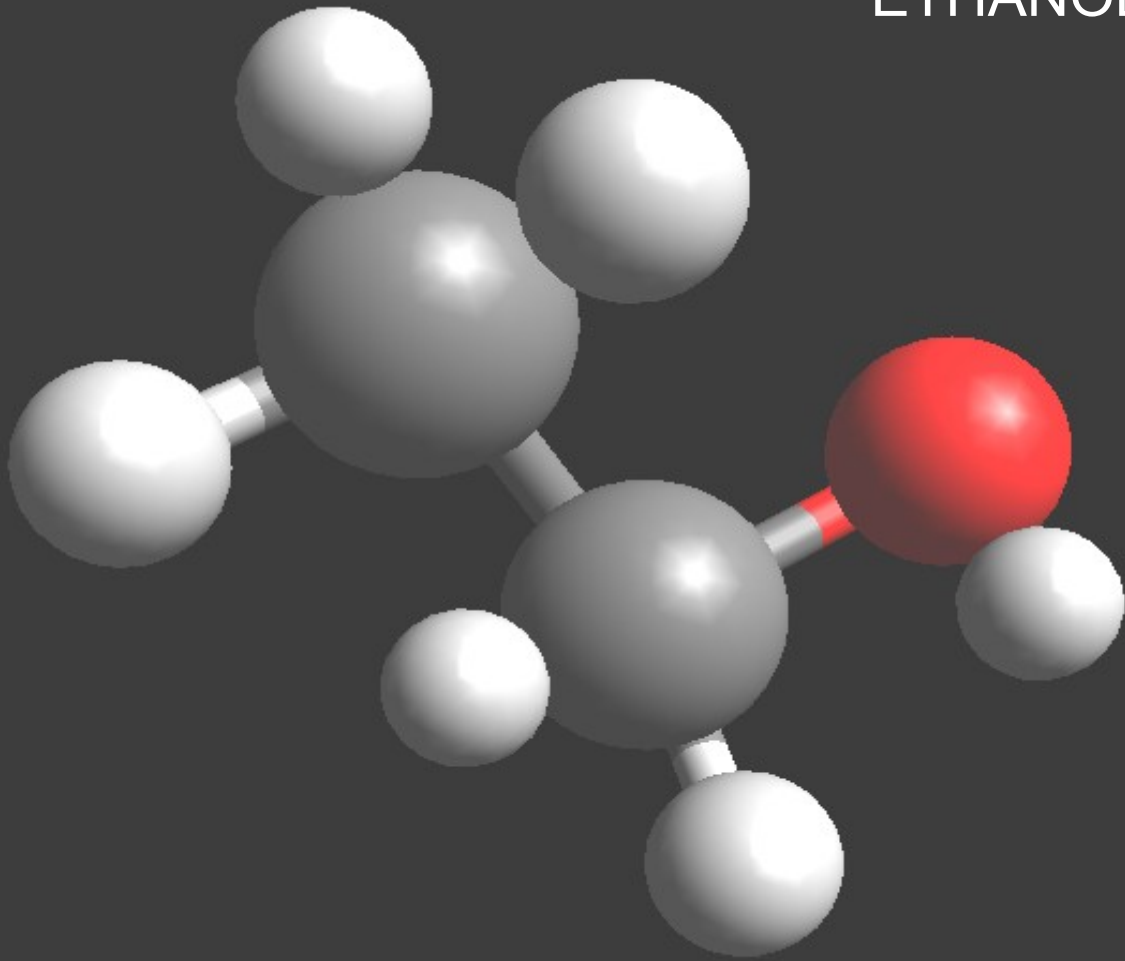
ÉTHANOL
