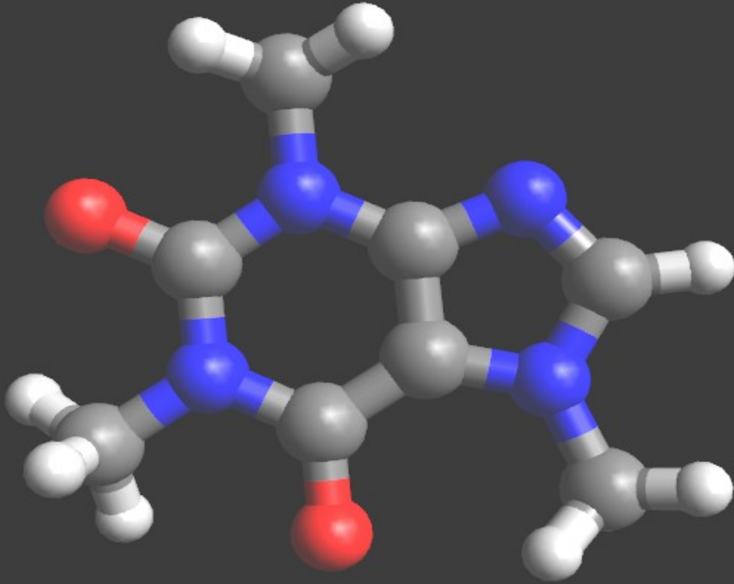
CAFÉÏNE
